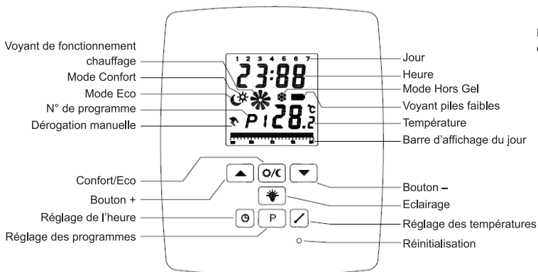
Figure 2. Emetteur
